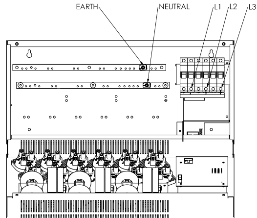
Einspeisung – Schukoversion
