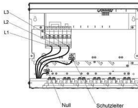
Anschlussdiagramm für die Versionen mit Ausgangsbuchsen (Schuko, UK etc.)
