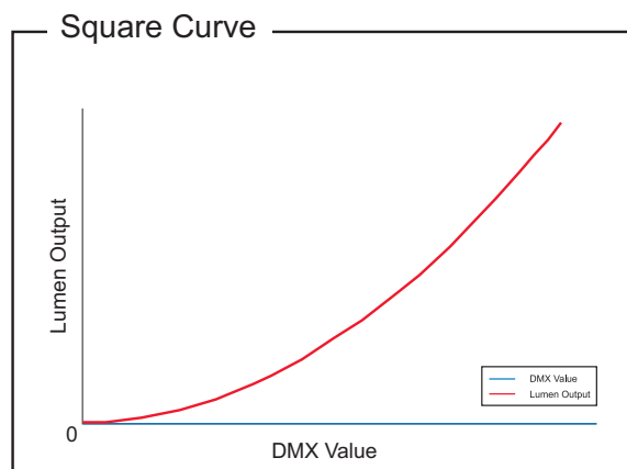
Figure 12: SL PAR 155 ZOOM RGBW LED Luminaire Dimmer Curves
